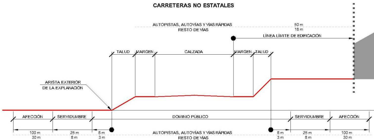
Fig.: Protección de carreteras (esquema orientativo)
