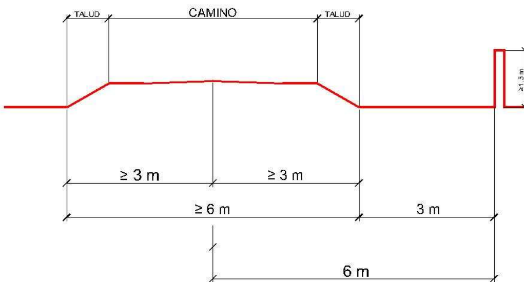
Fig: Protección de los caminos.
